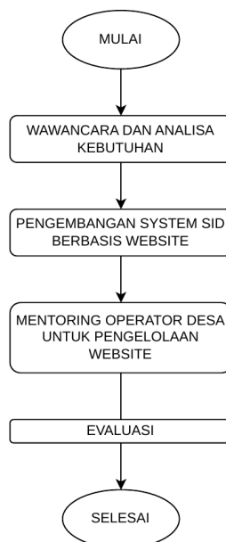
Gambar 1. Flowchart Kegiatan
